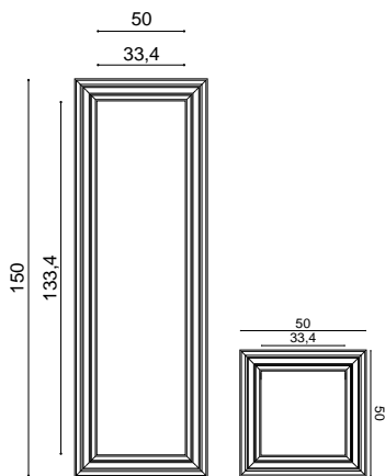
W120 + P4025 + W121 Purotouch® Дизайн Orio Tonini
