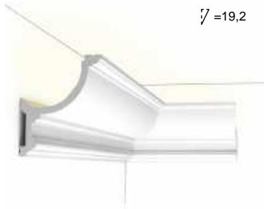
C901 | C901F Purotouch® 200 x 14,8 x 12,4 cm Дизайн Jacques Vergracht
